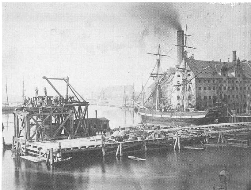
Mange tømrere var beskæftiget med arbejdet på den nye Knippelsbro 1868, selvom broen blev bygget af sten og jern. På billedet ses opførelsen af stillads til dykkerklokke. Fra tømrermester J. W. Unmack's fotoalbum. Københavns Tømmerlaug.
