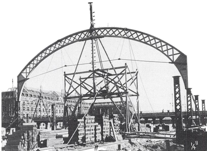
Fra opførelsen af Københavns hovedbanegård 1911. Perronhallernes gitterspær af træ var i forvejen samlede og blev hejset på plads ved hjælp af en tommerkonstruktion. Unmacks album, Københavns Tømmerlaug.
