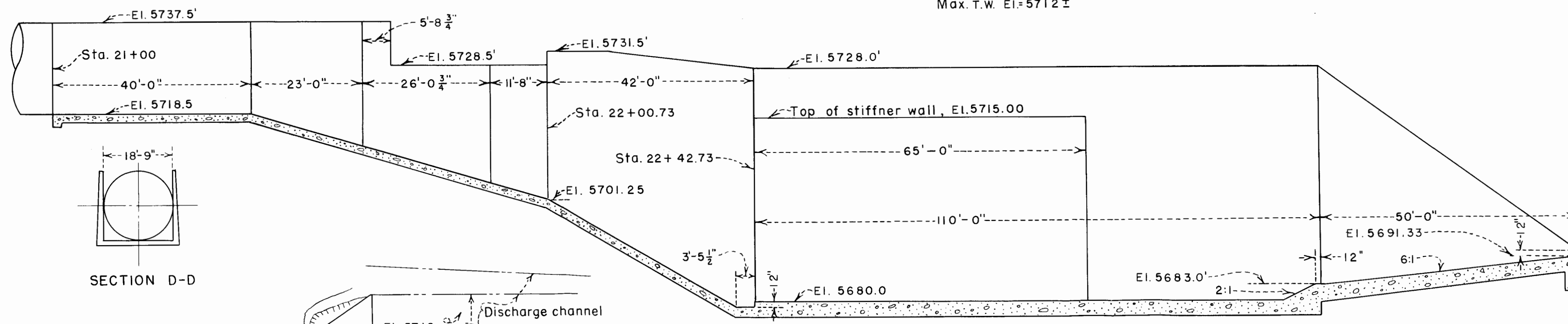
SECTION A-A
