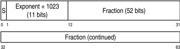
Figure 19-3. BFP Long Format (8 bytes)
