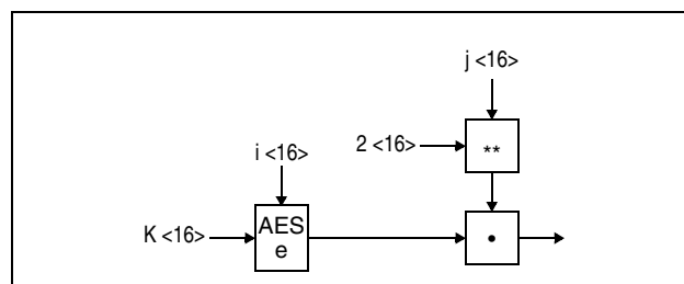
Figure 7-333. Compute XTS Parameter Using AES 128
