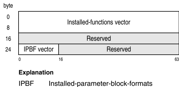
Figure 26-25. Parameter Block for DFLTCC-QAF
