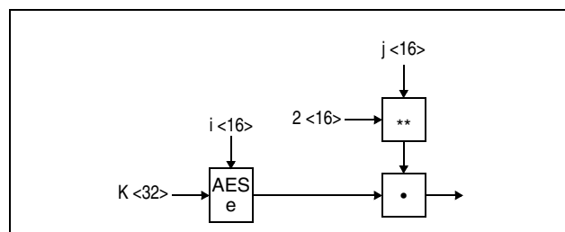
Figure 7-336. Compute XTS Parameter Using AES 256
