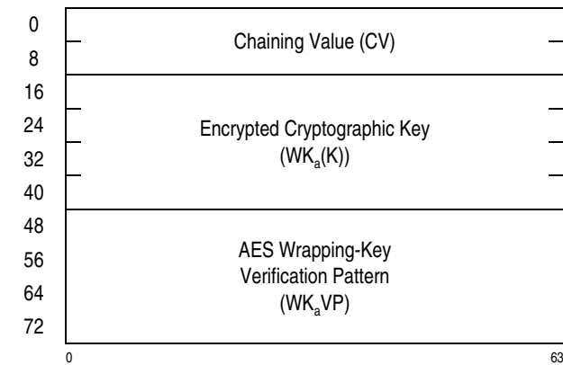
Figure 7-187. Parameter Block for KMO-AES-256
