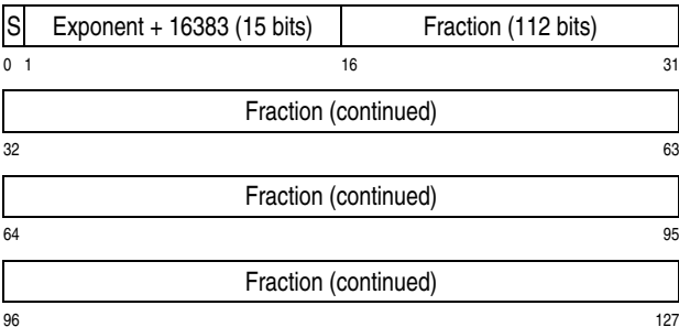
Figure 19-4. BFP Extended Format (16 bytes)
