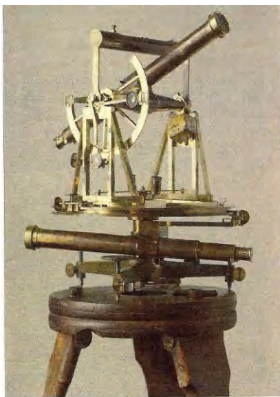
12zölliger Repetitionstheodolit von Reichenbach, Utzschneider und Liebherr, München um 1810
