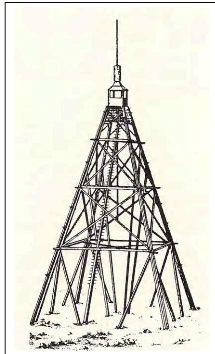
Bauart des ersten Turmes 1804 auf dem 520 Meter hohen Fuchsberg bei Johannesbrunn.
