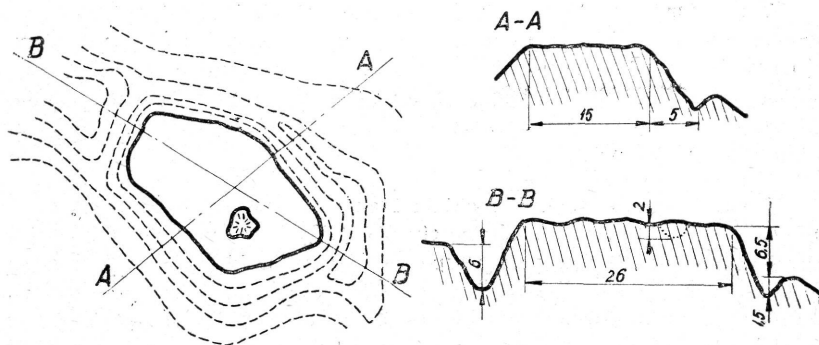
26. kép. A vár területe és metszete
