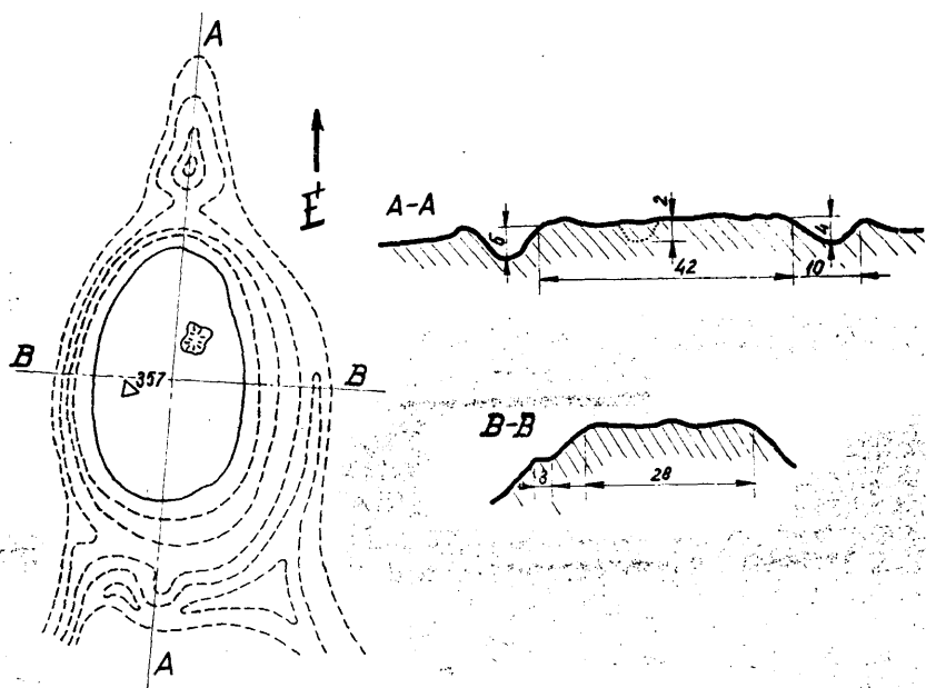
42. kép. A vár területe és metszete
